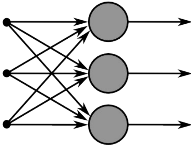
Einschichtiges Netz
