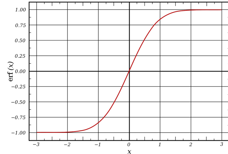
Sigmoidsche Aktivierungsfunktion
